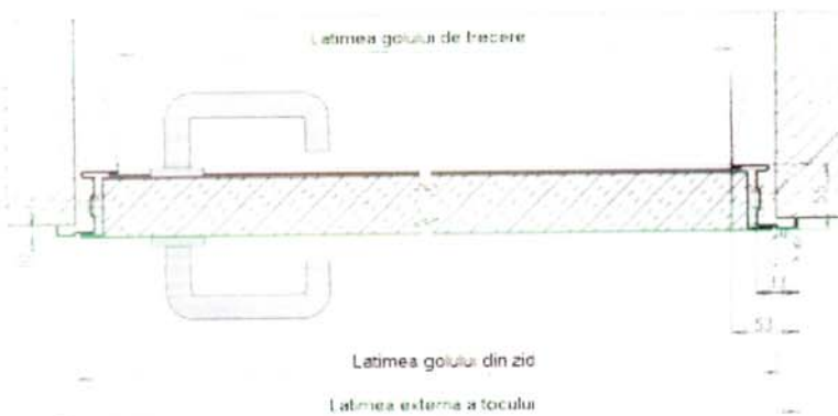
Fig. 2 - Ușă rezistentă la foc UNIVER
