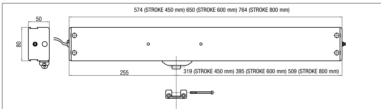
Actuators dimension
